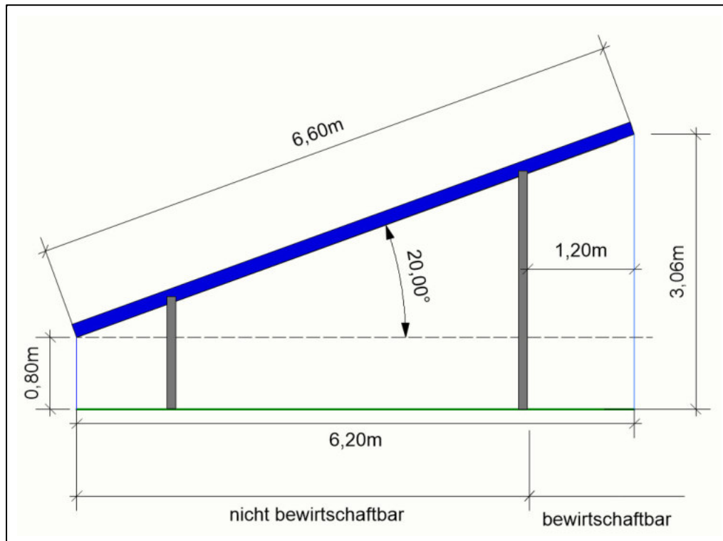
Abbildung 3: Modulschema
